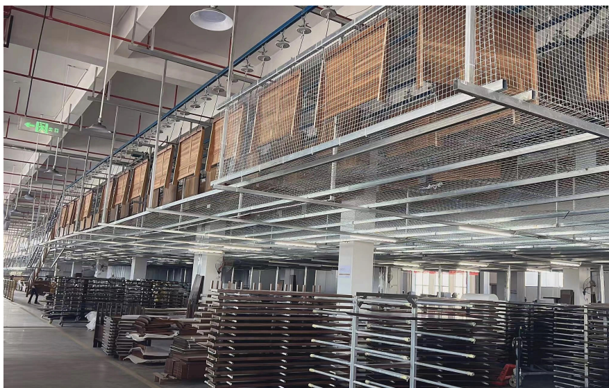
江西团团圆家具有限公司的吊线喷房生产线高速运转
